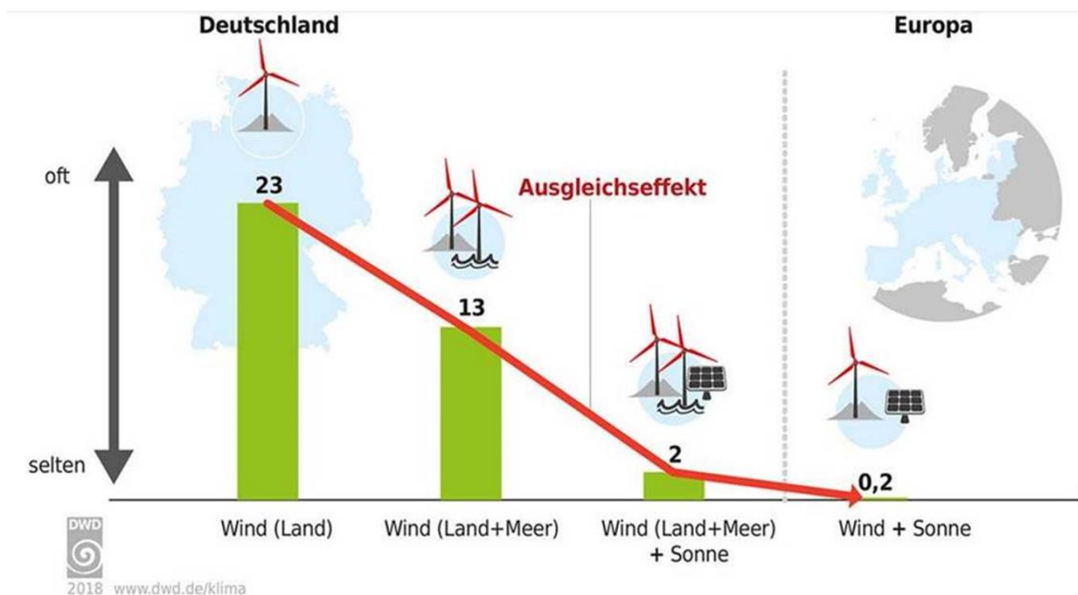
Abbildung 10: Verteilung erneuerbarer Kapazitäten im europäischen Stromverbund mindert Ertragsausfälle von erneuerbaren Energien
