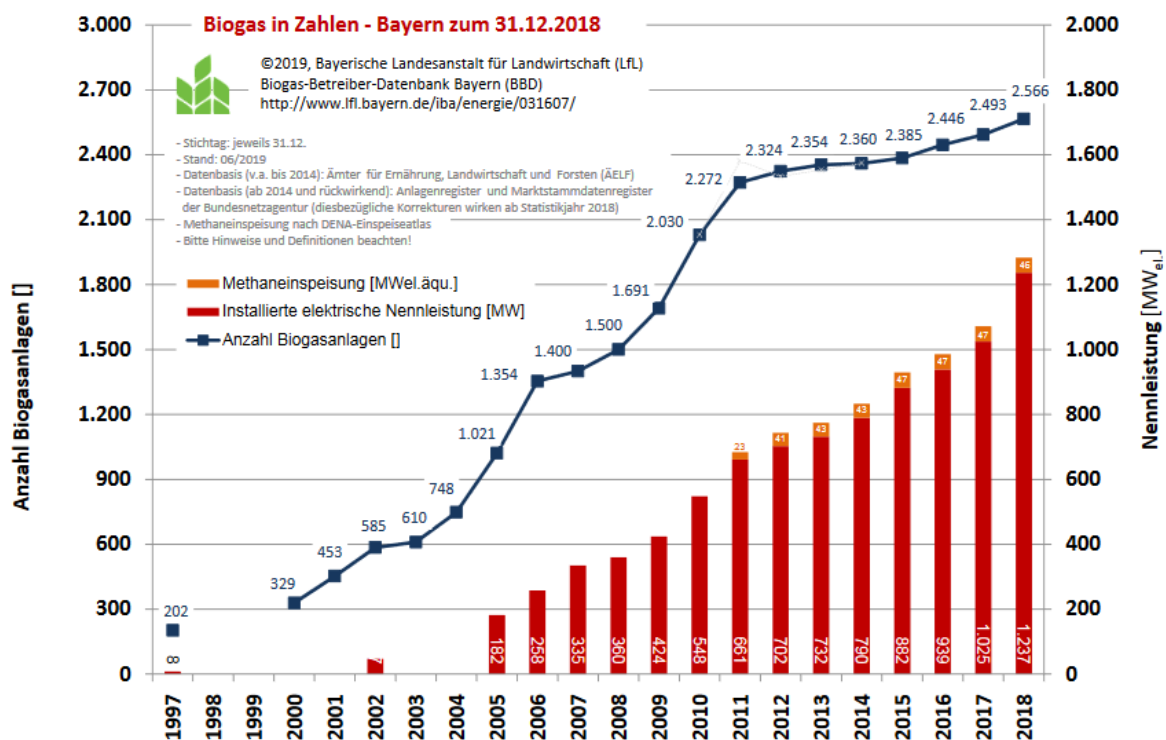
Abbildung 7: Installierte elektrische Leistung von Biogasanlagen in Bayern
