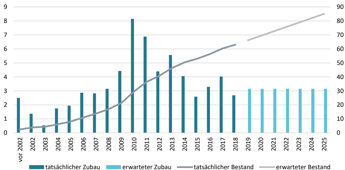
Abbildung 3: Jährlicher PV-Zubau und Bestand in München (MW) mit Fortschreibung bis 2025
