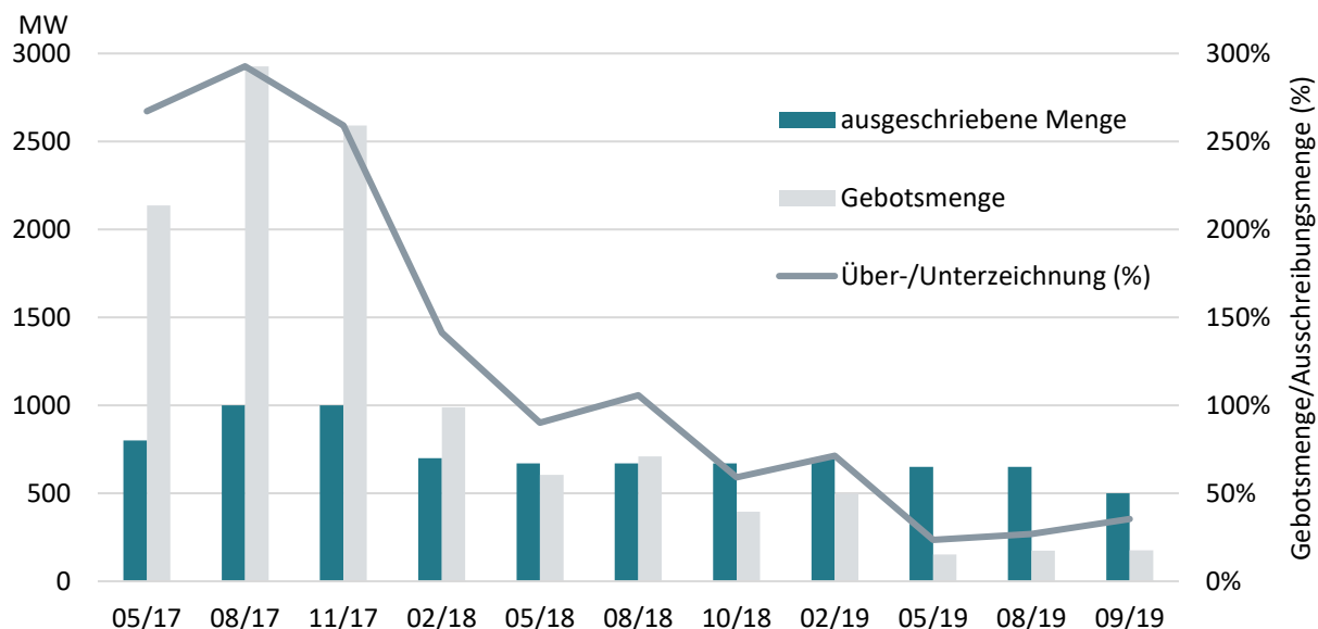
Abbildung 6: Über-/Unterzeichnung der Ausschreibungsmengen Onshore-Wind
