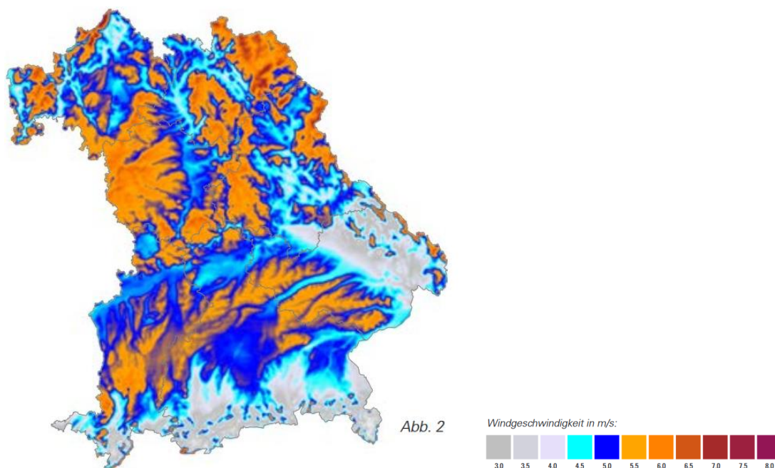
Abbildung 4: Windgeschwindigkeit in 130 m Höhe über Grund
