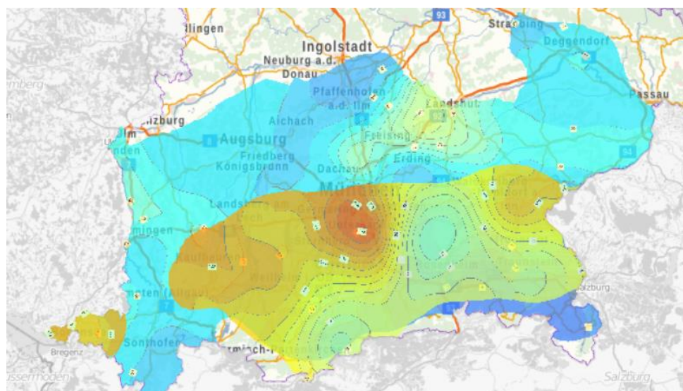
Abbildung 8: Temperaturverteilung im südlichen Bayern (blau hervorgehoben) in 3000m Tiefe
