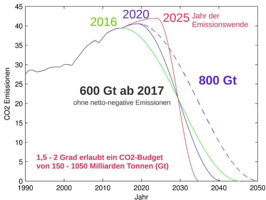
Abbildung 9: Globales Treibhausgasbudget und Emissionspfade
