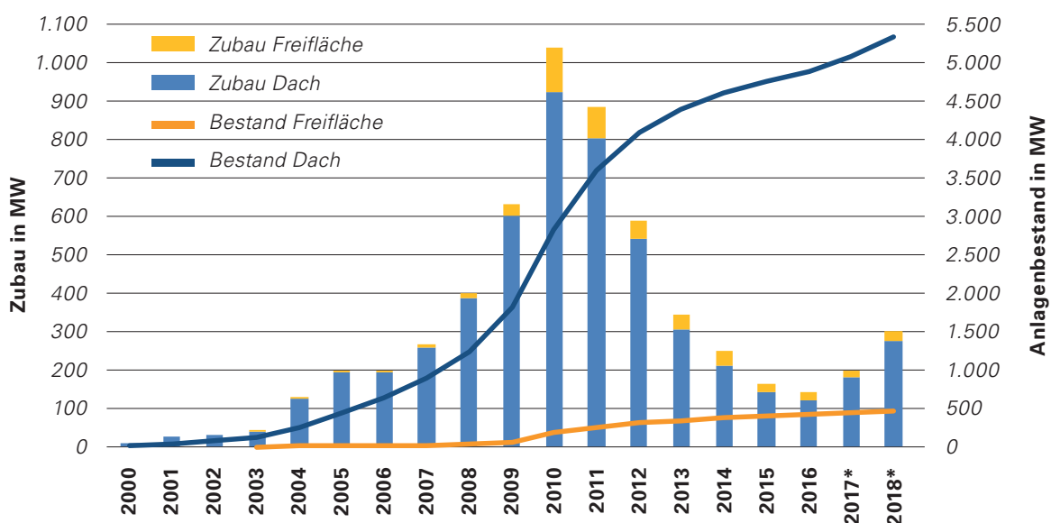
BILD 1: ENTWICKLUNG VON ZUBAU UND BESTAND VON PHOTOVOLTAIKANLAGEN IN BADEN-WÜRTTEMBERG.
