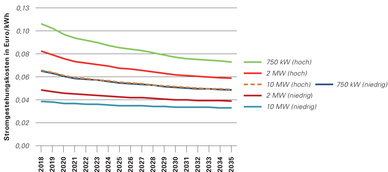
BILD 5: STROMGESTEHUNGSKOSTEN FÜR ZUKÜNFTIGE ANLAGEN. DIE GRAFIK ZEIGT JEWEILS DEN WERT FÜR NEUE ANLAGEN IM SPEZIFISCHEN JAHR.
