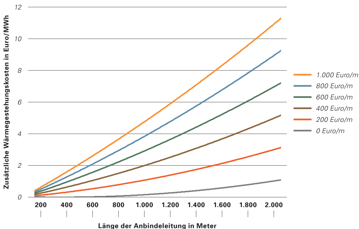
BILD 14: MEHRKOSTEN FÜR DIE WÄRMEGESTEHUNG FÜR EINE ANLAGE MIT 30.000 m 2 KOLLEKTORFLÄCHE IN ABHÄNGIGKEIT VON DER DISTANZ ZUM EINBINDEPUNKT SOWIE DEN SPEZIFISCHEN KOSTEN FÜR DIE ANBINDELEITUNG.
