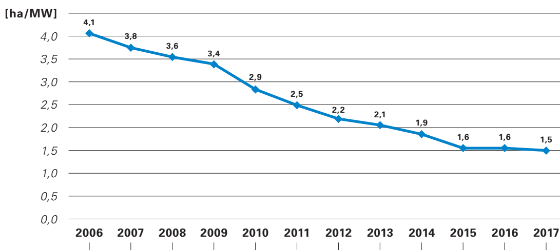
BILD 4: ENTWICKLUNG DER SPEZIFISCHEN FLÄCHENINANSPRUCHNAHME IN ha/MW VON NEUEN PHOTOVOLTAIK-FREIFLÄCHENANLAGEN IN DEUTSCHLAND.
