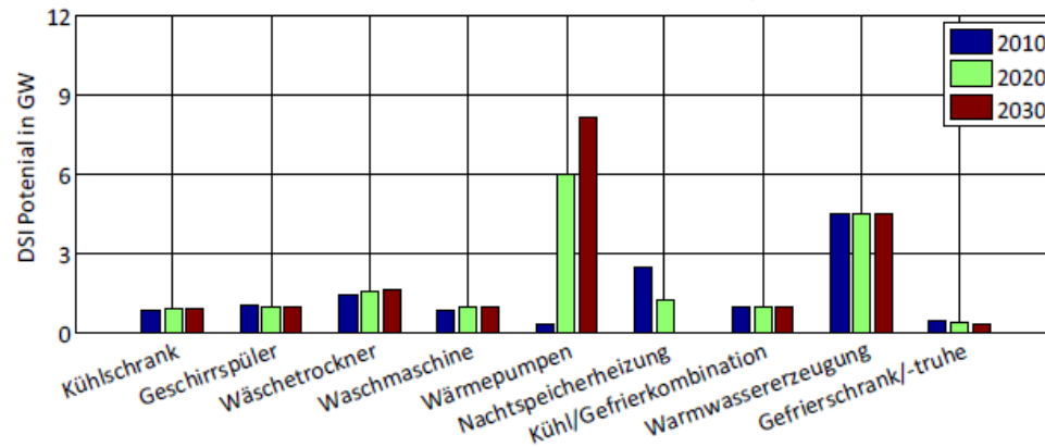
Theoretisches DSI Potential im Bereich Haushalt, Winterfall
