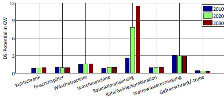
Theoretisches DSI Potential im Bereich Haushalt, Sommerfall
